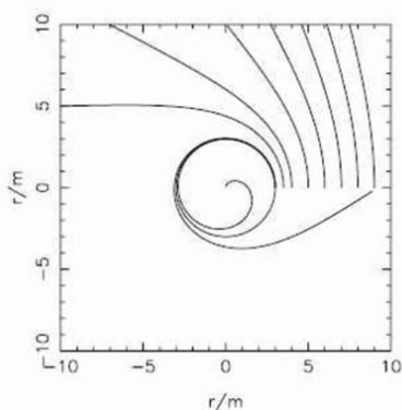
Fig. 1 (Desviación del fotón cerca de un objeto con una masa pesada) 1
