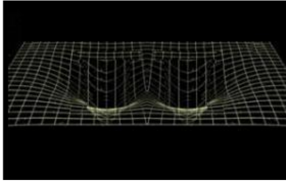
Ilustración 1.2. Representacion de curvaturas 2 partículas db 2
